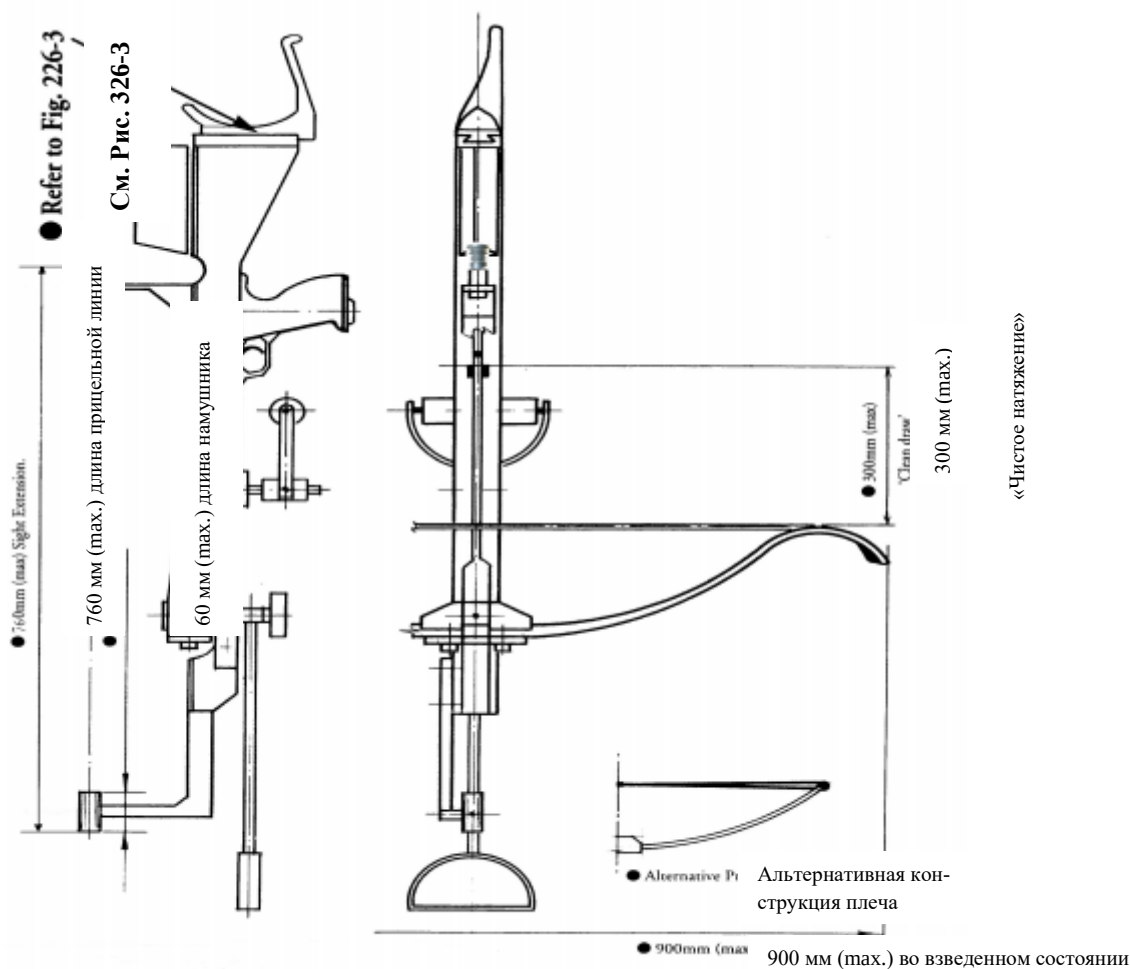
Рис. 326-1: Характеристики арбалета (см. Ст. 326.5.1)
