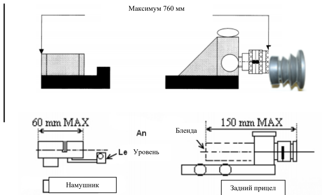
Рис. 326-2: Ограничения для прицелов
