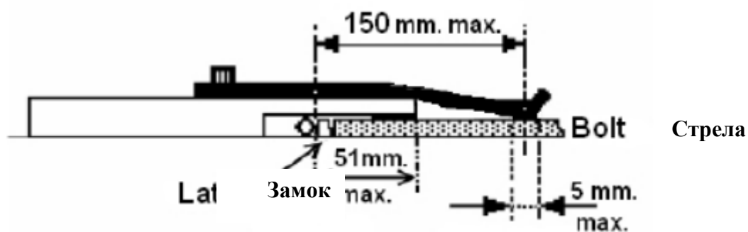
Рис. 326-4: Ограничения для фиксаторов стрел и направляющей тетивы
