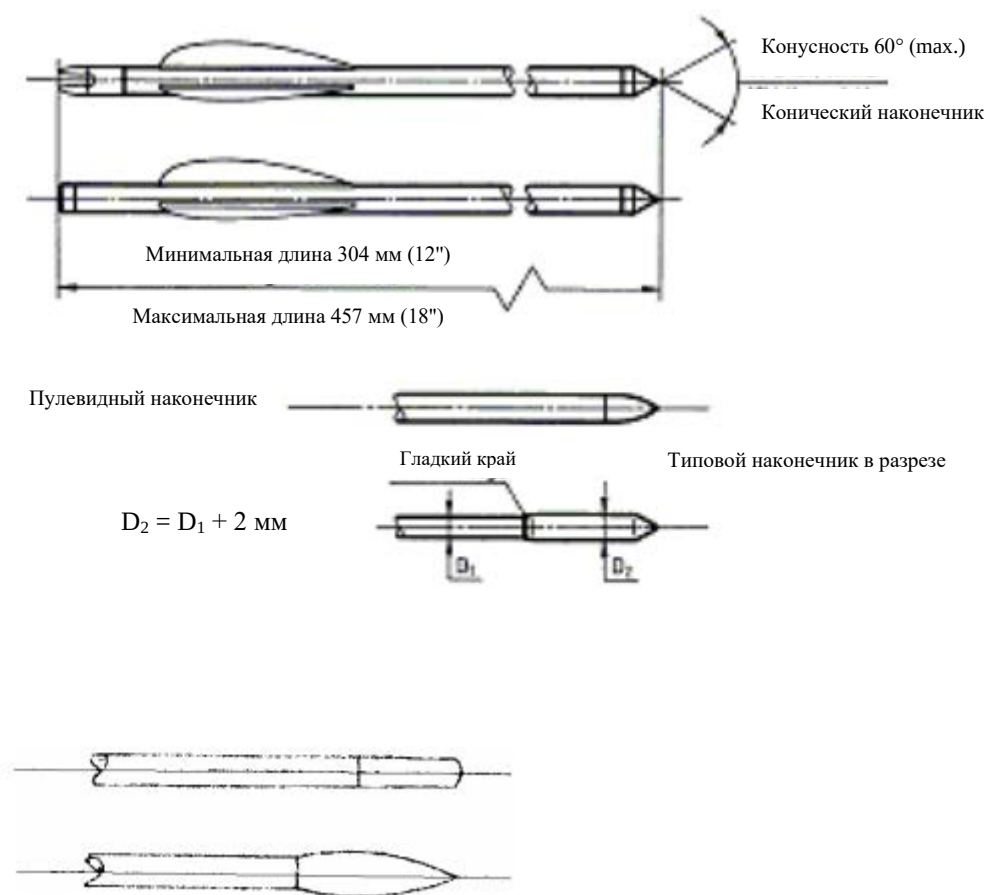
Рис. 327.1: Характеристики стрел (см. Ст. 327)
